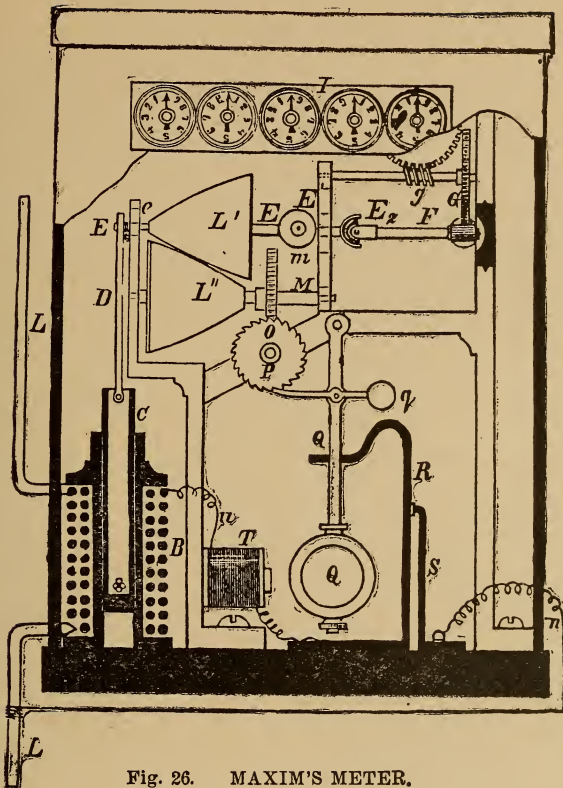
Fig. 26. MAXIM'S METER.
